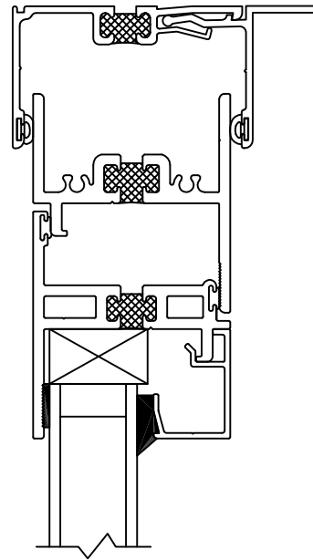
#8124-RECEPTOR #8128-FLANGE CLIP
