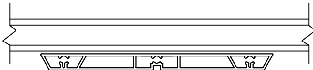
#9064 MUNTIN
